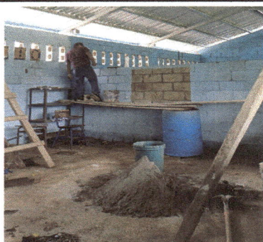
Foto.14. Construcción de muro de mampostería en un módulo de aula.
