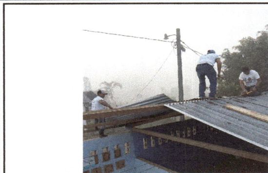
Foto 1. Retiro de láminas acanaladas, en los tres módulos de aulas, trabajo previo a instalar láminas troqueladas.
